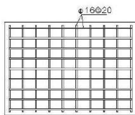
پلان فنداسیون بستر پمپ آتش نشانی نمای تحتانی
